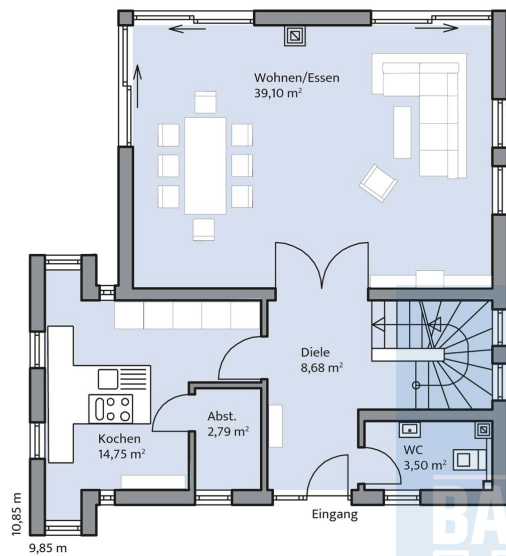
Haus Haas Grundriss
