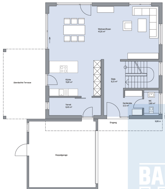
Haus Kersten Grundriss
